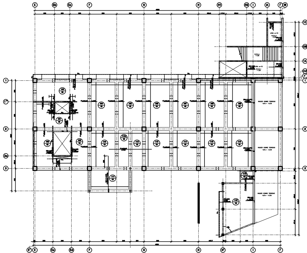
ARMADURA MALLA SUPERIOR LOSA CIELO 1° PISO
